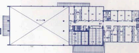
3階平面図
